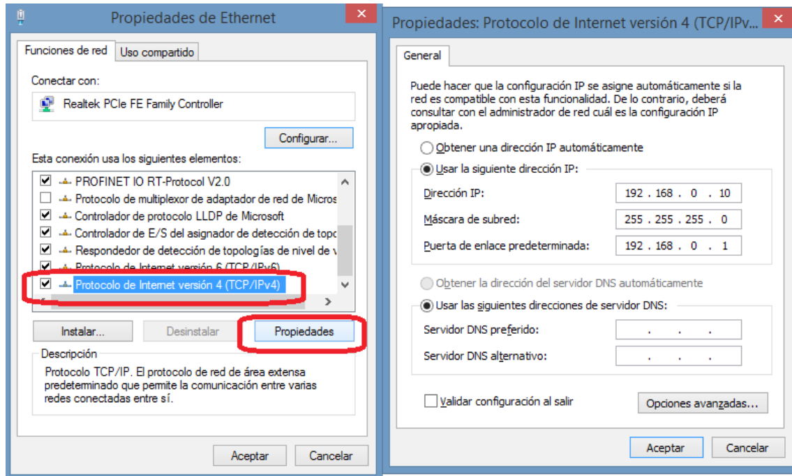
Figura 30. Dirección IP, máscara de subred y puerta de enlace predeterminada de la PC.
