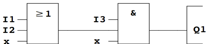
Figura 5. Bloque OR.
